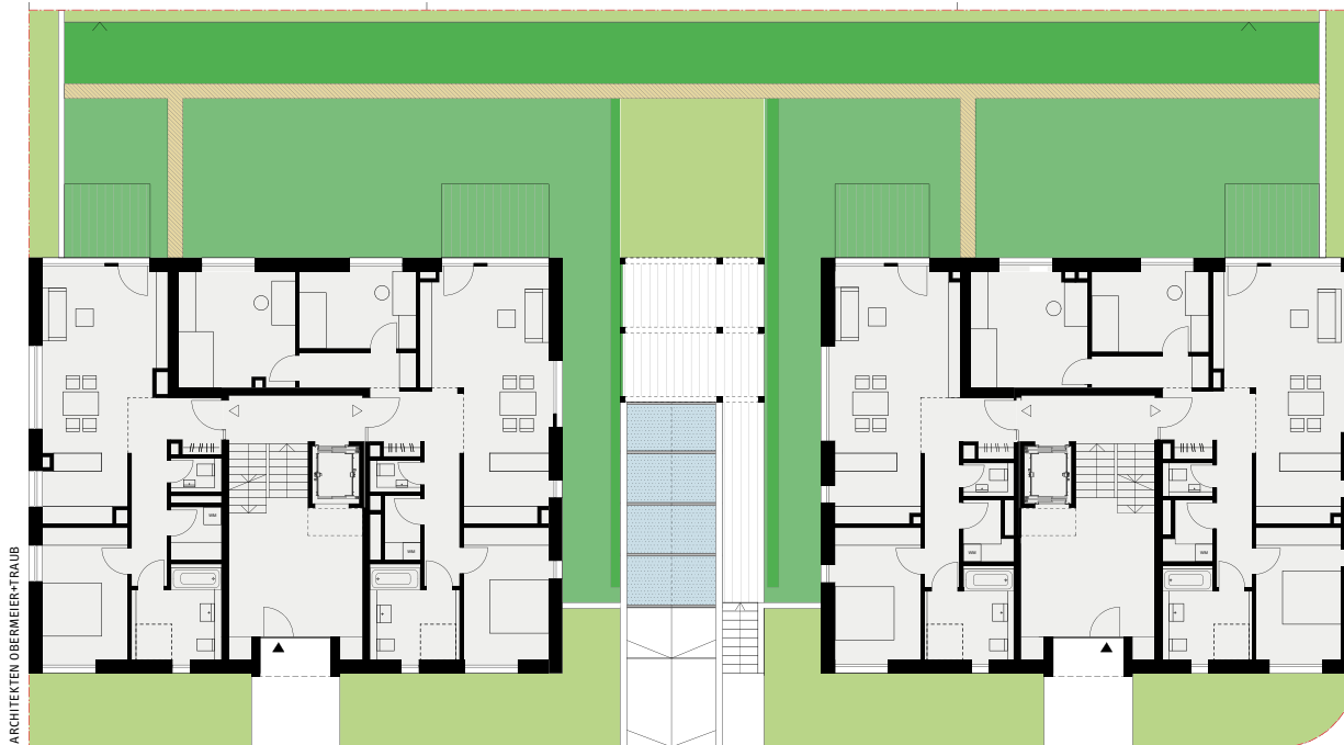
ERDGESCHOSS Die baugleichen Fünfgeschosser sind in der Mitte verbunden.
